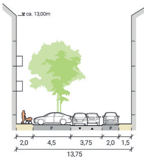
Abb. 18 (links): Querschnitt Klauprechtstraße im Szenario ‚Trend‘. In Grün- derzeitquartieren fehlen oft bequem erreichbare, sichere Fahrradabstelan- lagen.
