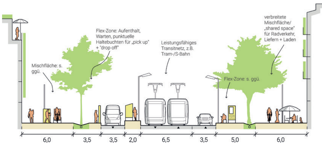
Abb. 16: Querschnitt Kaiserallee im Szenario ‚Sharing‘
